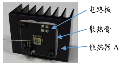
照片 2 评价光源的散热结构
