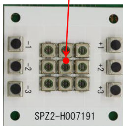
照片 4 安装状态
