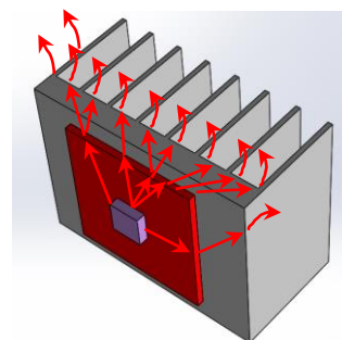
图 5 让鳍片向侧面设置时的 散热路径示意图
