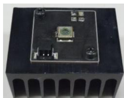
照片 9 让鳍片向下设置 (妨碍空气流动的朝向)
